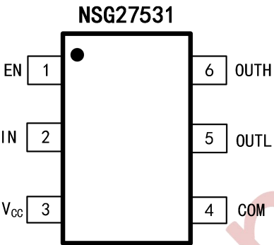
图 6-1 SOT23-6 顶视图
