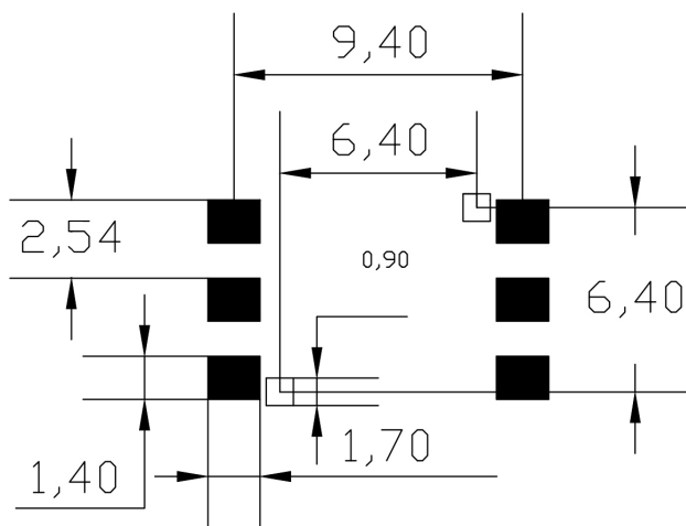
图 9. 建议焊盘图
