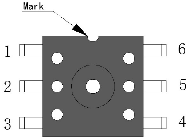
图 1. 引脚配置图
