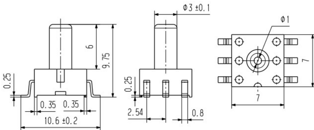
图 8. 产品尺寸图
