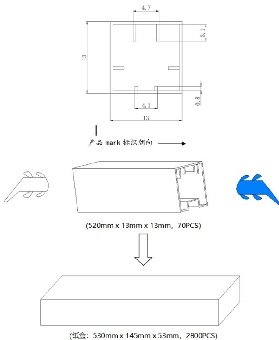
图 12. 料管图纸
