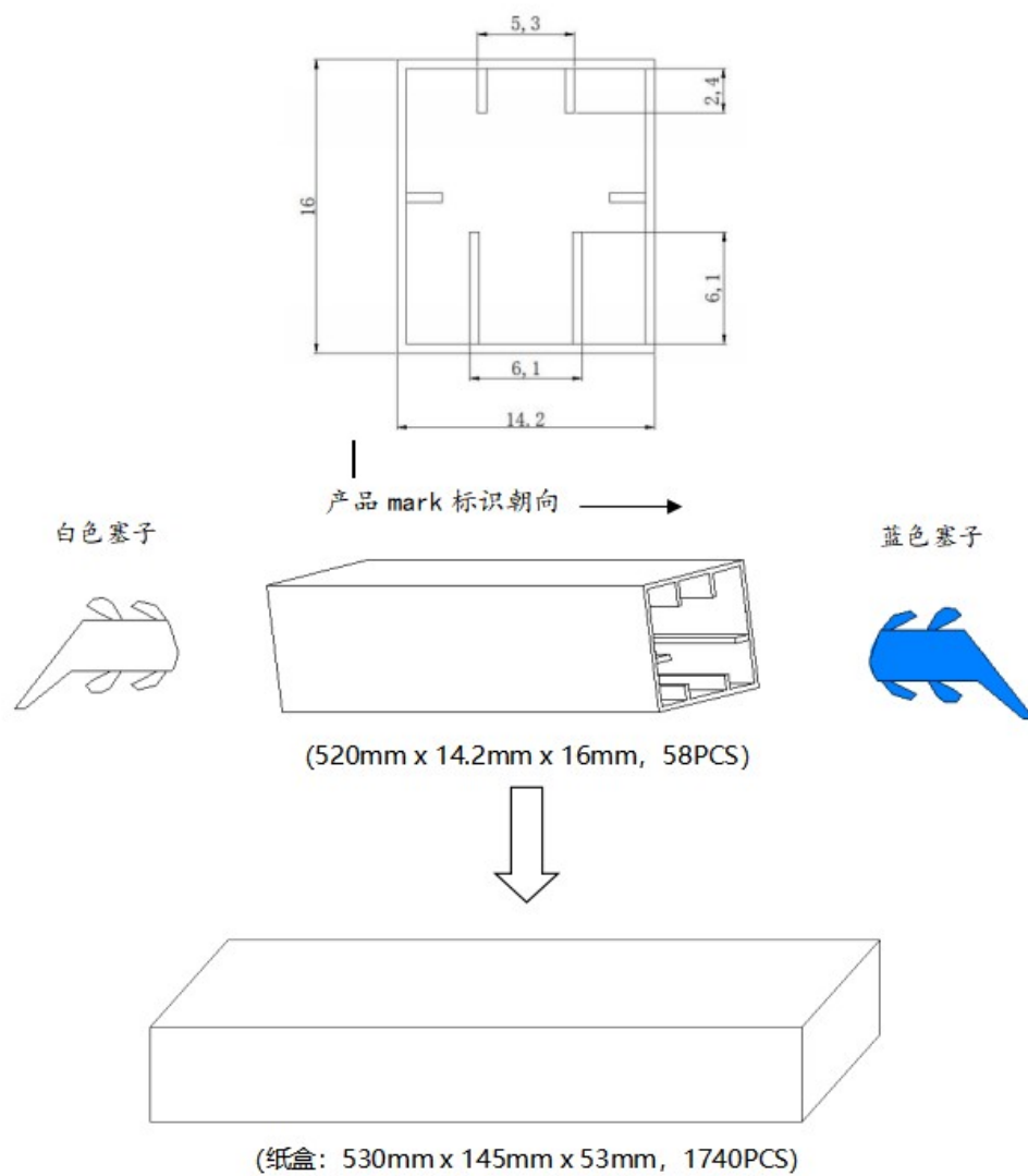
图 12. 料管图纸
