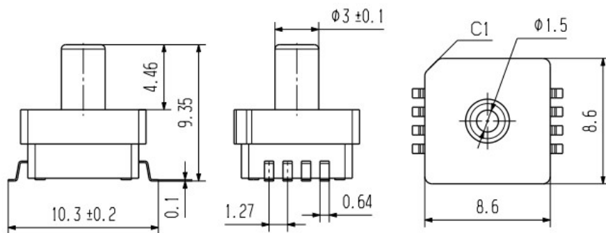
图 8. 产品尺寸图
