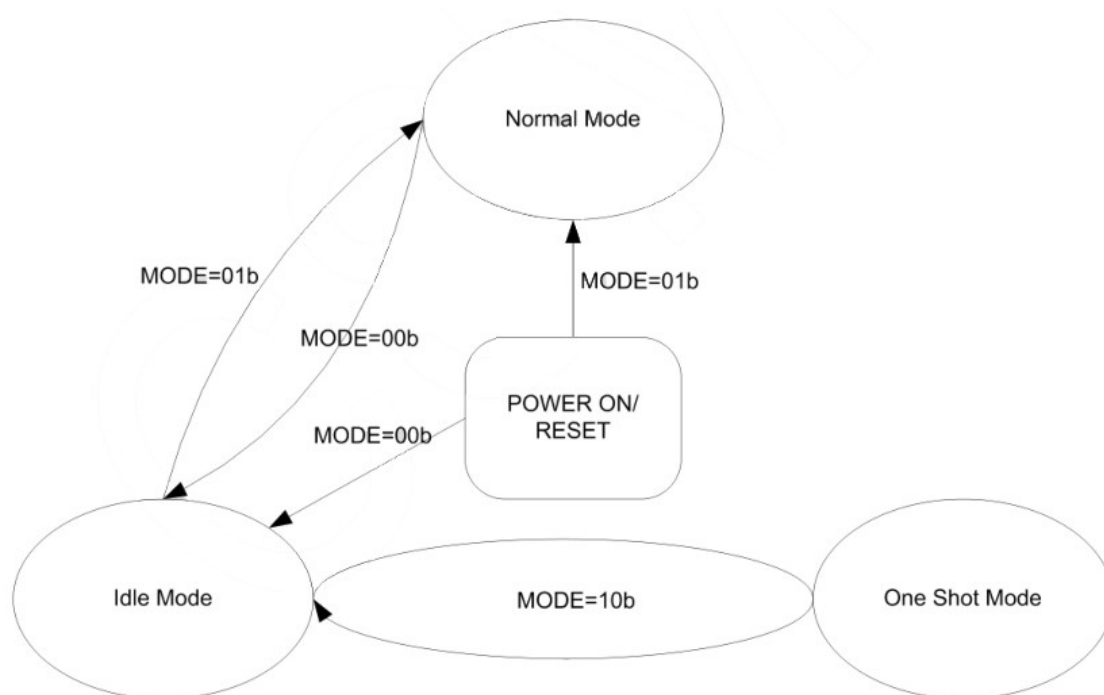
图 7. 工作模式转换流程图
