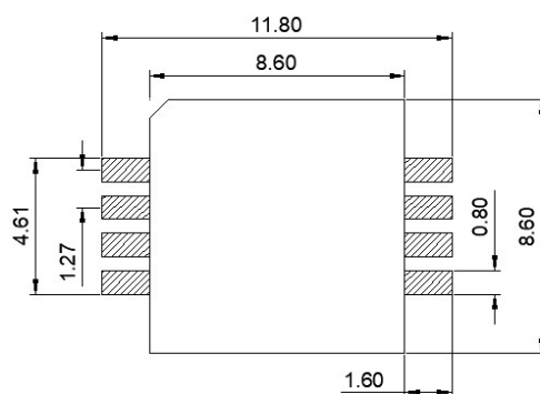
图 10. 建议焊盘图
