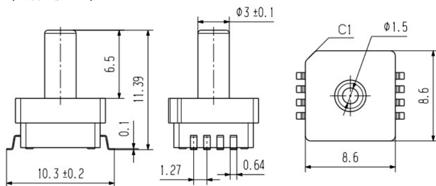
图 9. 产品尺寸图
