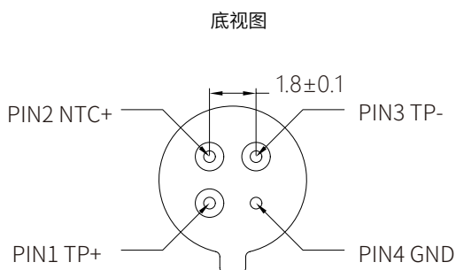
电气连接
