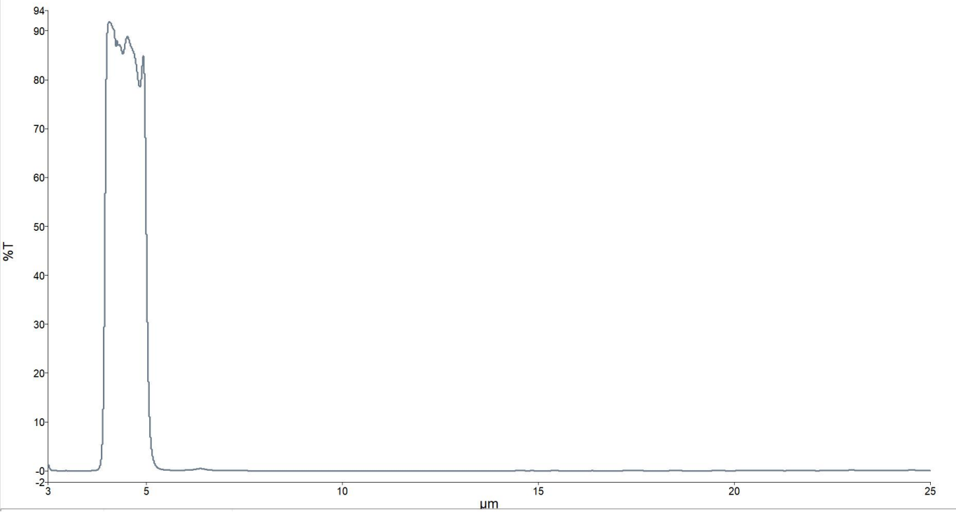
附：1. 光谱图
