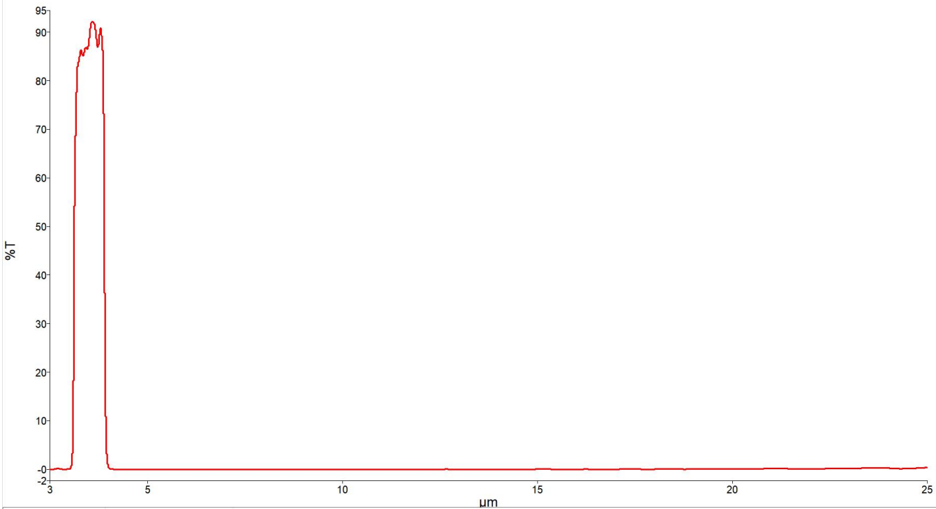
附：1. 光谱图
