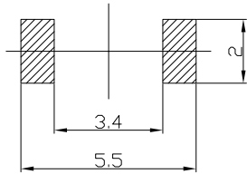
安装参考尺寸
