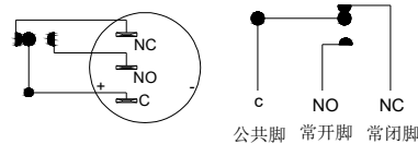
No electrical schematic diagram 无灯电气原理图
