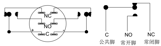
Electrical principles without lights 无灯电气原理
