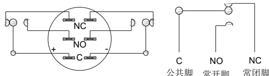
Electrical principles without lights 无灯电气原理
