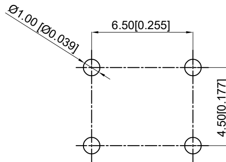
PCB. Welding diagram PCB.焊接图
