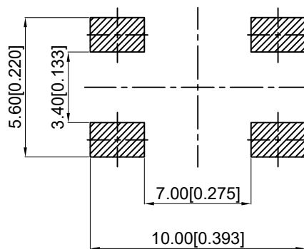
Welding diagram 焊接图
