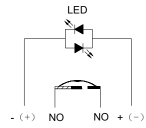
Schematic Diagram 电气原理图
