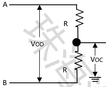
图 1 驱动器直流特性测试负载
