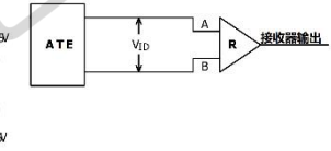
图 9 接收器传输延时测试
