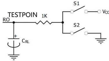
图 2 接收器使能/关断 开关特性测试负载
