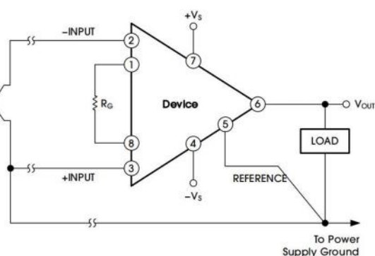
热电偶输入时的偏置电流接地回路
