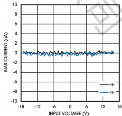
输入偏置电流与共模电压 (25°C)
