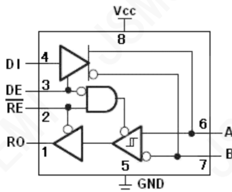
图2: MAX13085EESA-JSM逻辑图
