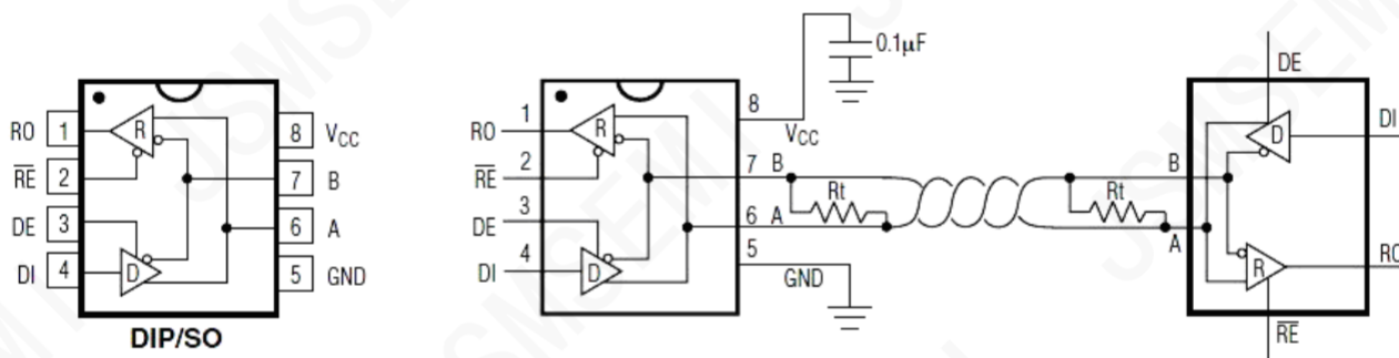
图 3: MAX13085EESA-JSM典型半双工应用电路
