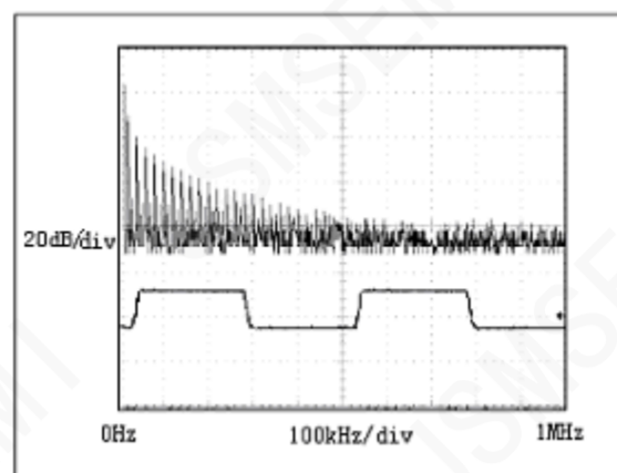
图 13: 传输 20kHz 信号时 MAX13085EESA-JSM驱动器输出 波形和 FFT 图
