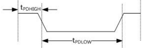
图 11.9 时隙图
