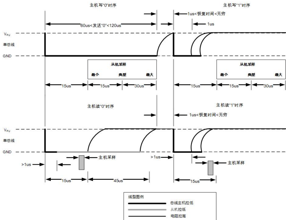
图 11.6-2 读/写时序
