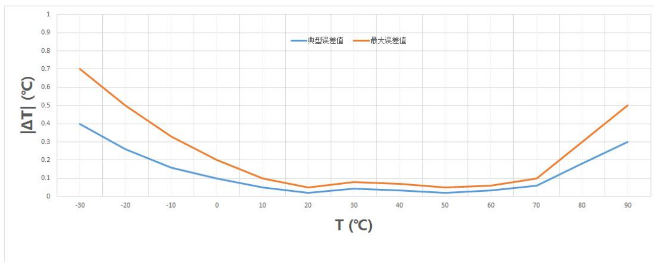
图 7-1 T1601Z 精度误差曲线
