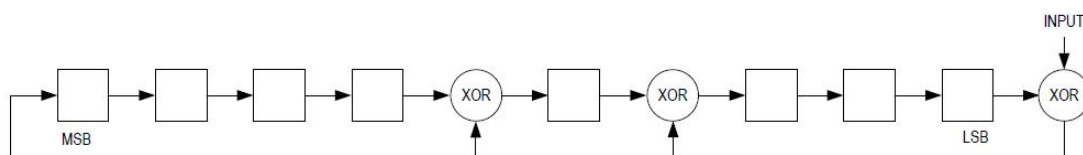
图 9.5 CRC 发生器
