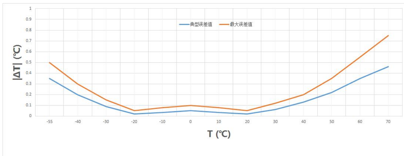
图 7-3 T1601P 精度误差曲线
