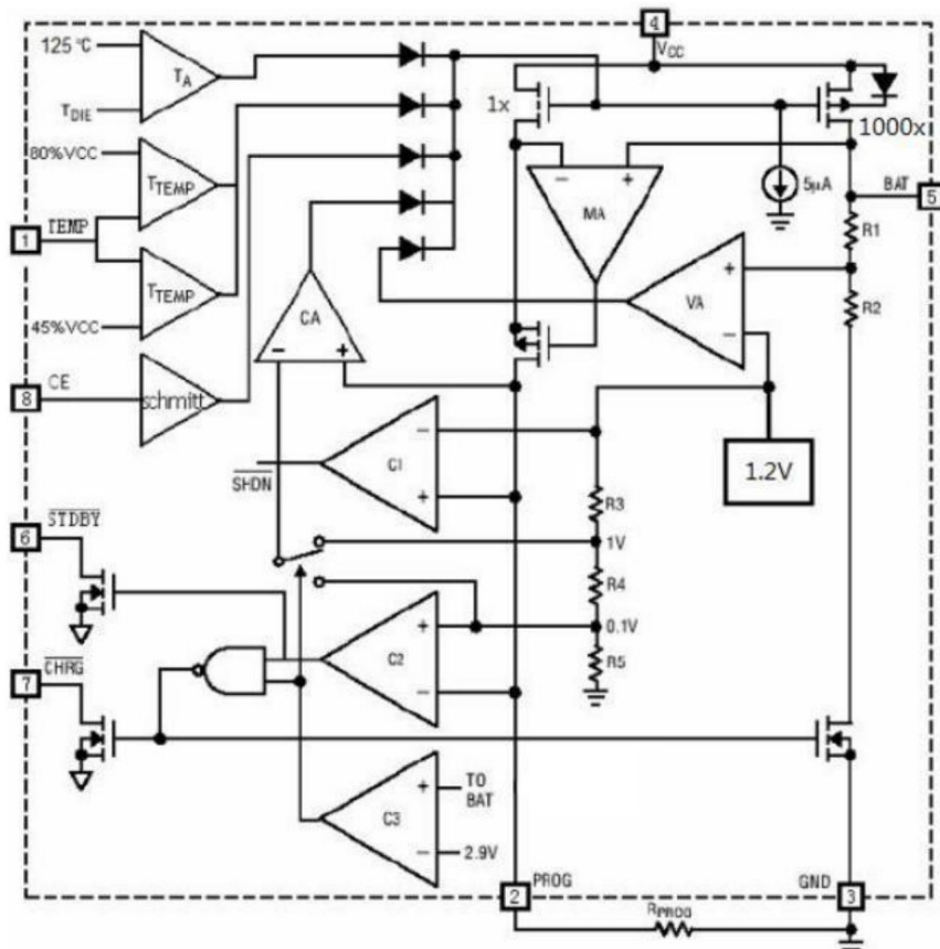
内部结构图
