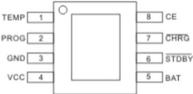
Fig3 管脚示意图
