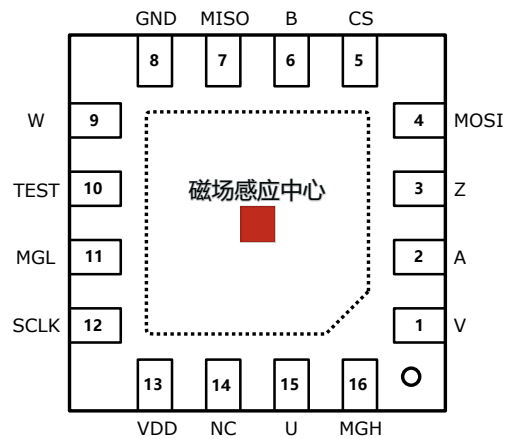
图 3: QFN-16L 3mmx3mm
