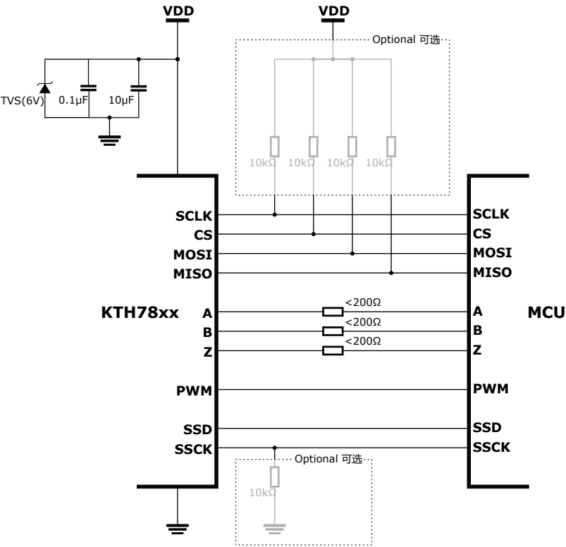
图 2: 应用电路
