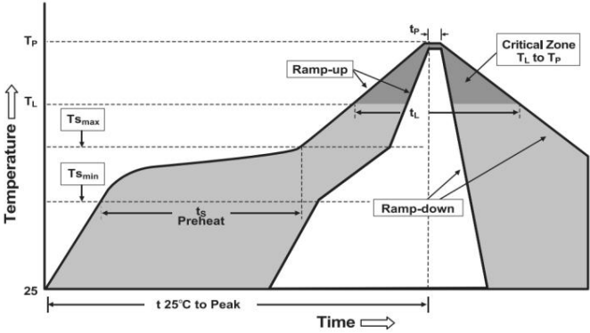
Soldering Parameters/焊接参数
