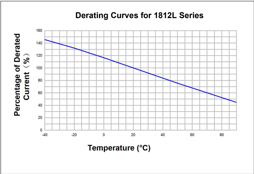
Thermal Derating Curve/环境温度与工作电流关系特性图
