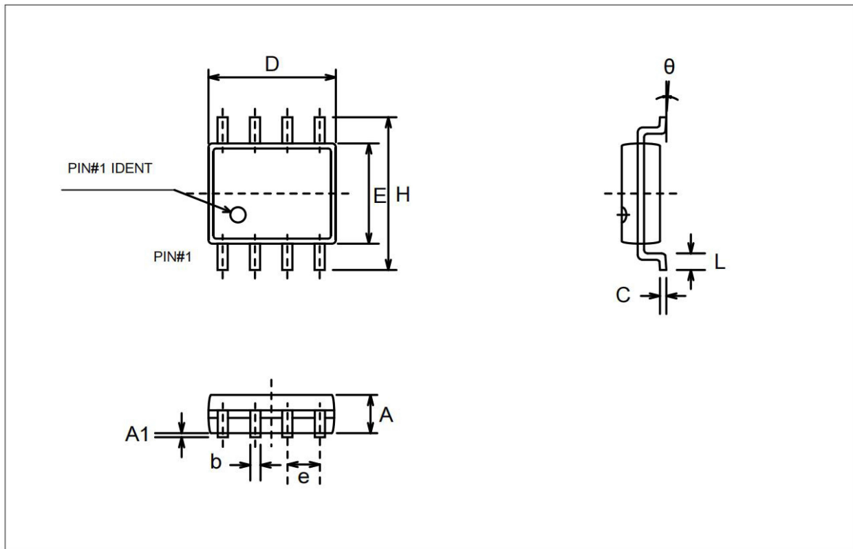
图 4-1: SOP8封装示例
