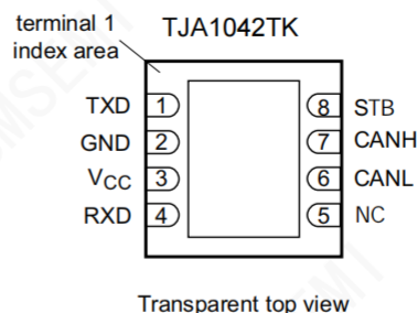
b. TJA1042TK: SOP-8
