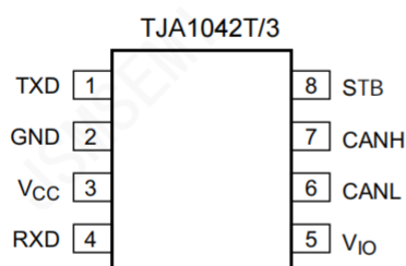
c. TJA1042T/3: SOP-8
