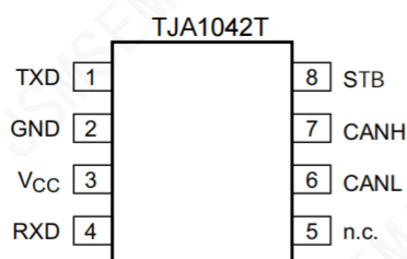
a. TJA1042T: SOP-8
