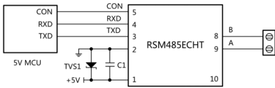
图3.MCU 5V供电应用电路
