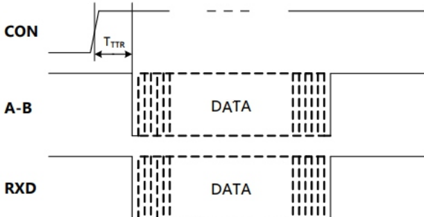
图2. RSM(3)485ECHT模块数据接收时序图
