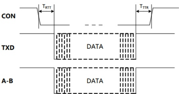
图1. RSM(3)485ECHT模块数据发送时序图
