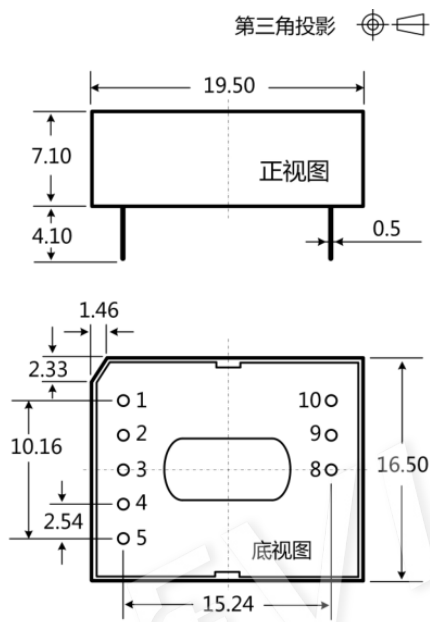
外观尺寸图
