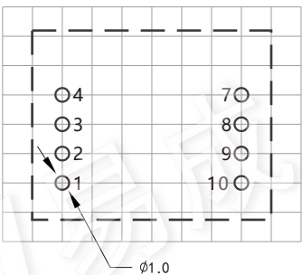
建议印刷图
