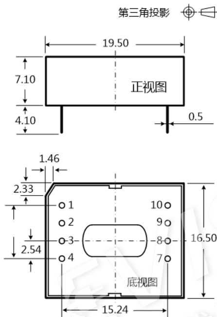
外观尺寸图
