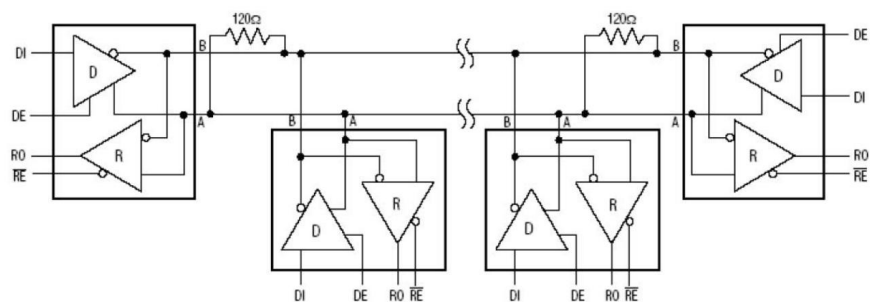
图13: 典型半双工RS-485网络
