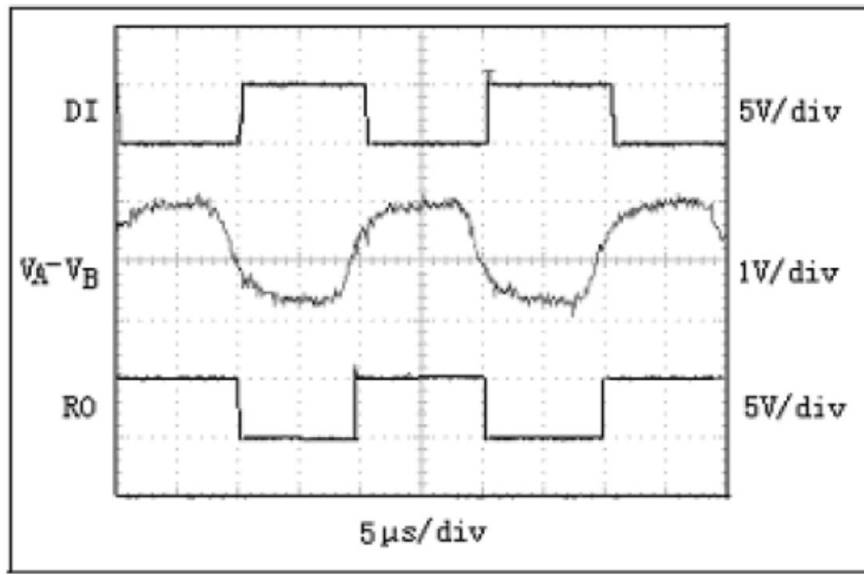
图 12: 在 50kHz 时驱动 4000 英尺的电缆
