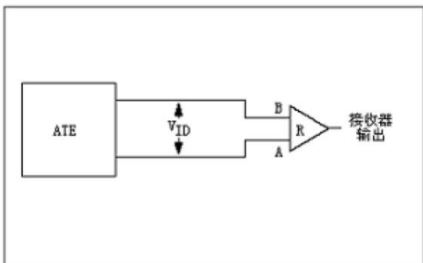
图 10:接收器传播延时测试电路
