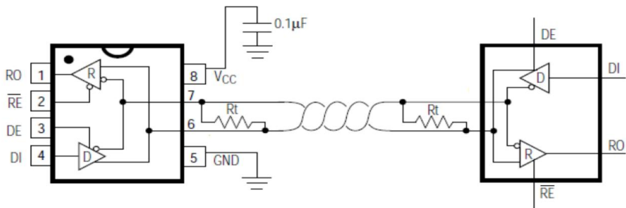
图 1: VP3085 典型半双工应用电路
