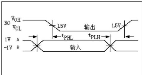
图 8:接收器传播延时
