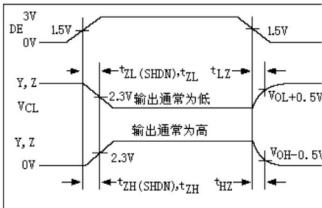
图 7:驱动器使能和无效时间
