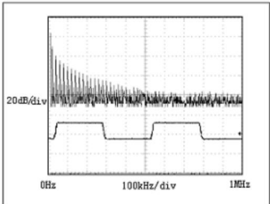
图 11:传输 20kHz 信号时 VP3085 驱动器输出波形和 FFT 图
