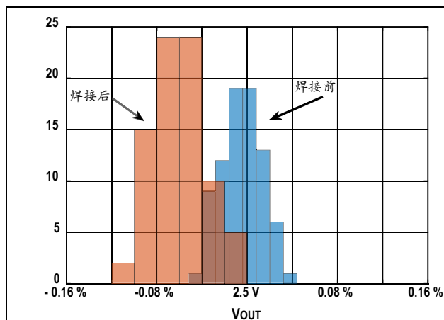
图22. ADR431 SOIC8 封装芯片焊接前后电压分布图
