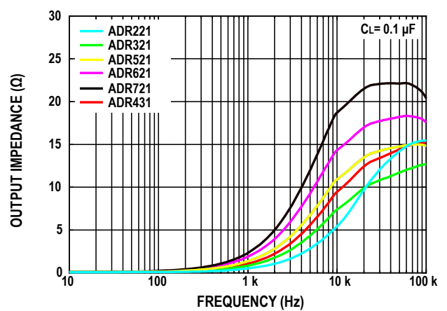
图13. 输出阻抗与频率的关系
