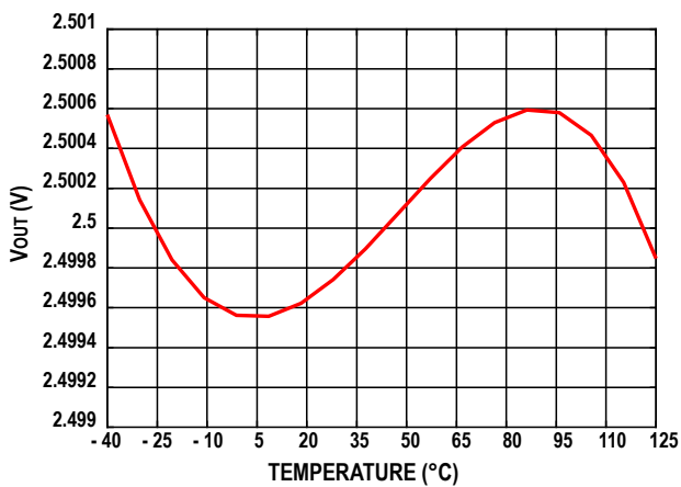
图4. ADR431 典型输出电压与温度关系
