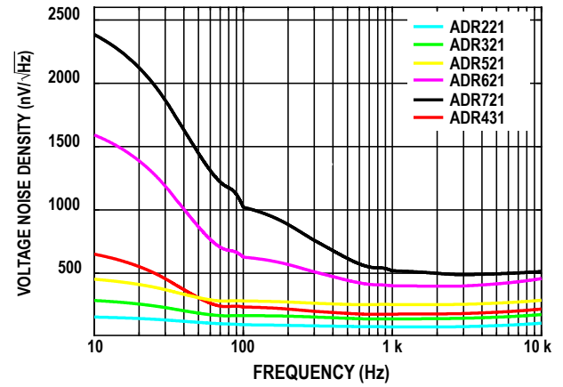
图11. 输出电压噪声 (10 Hz 至 10k Hz)
