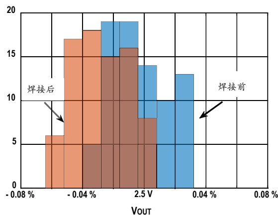
图23. ADR431 MSOP8 封装芯片焊接前后电压分布图
