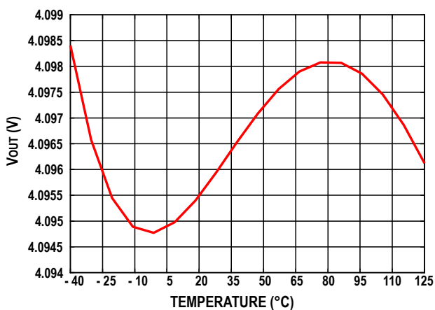
图6. ADR621 典型输出电压与温度关系
