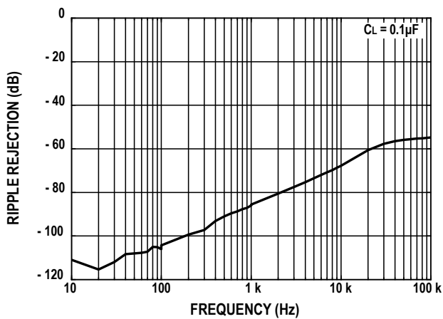
图12. ADR441 电源抑制比与频率的关系
