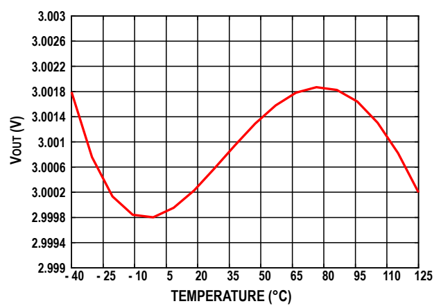
图5. ADR521 典型输出电压与温度关系
