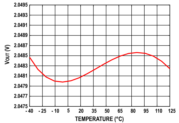
图3. ADR321 典型输出电压与温度关系
