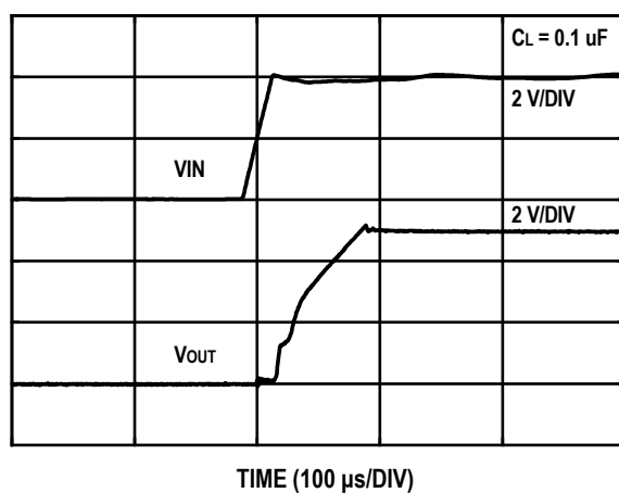
图15. ADR431 开启响应
