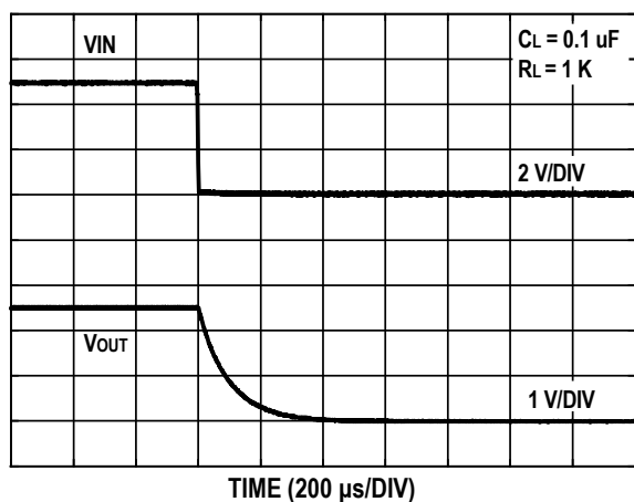
图14. ADR431 关闭响应
