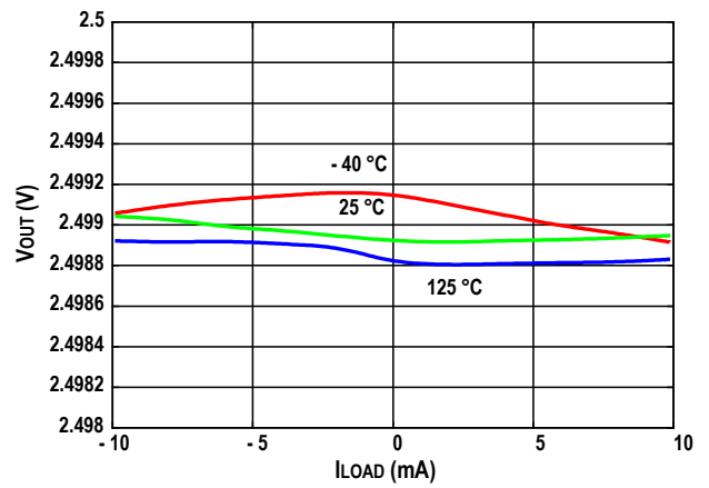
图9. ADR431 负载调整率
