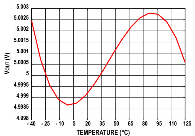
图7. ADR721 典型输出电压与温度关系
