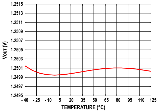
图2. ADR221 典型输出电压与温度关系
