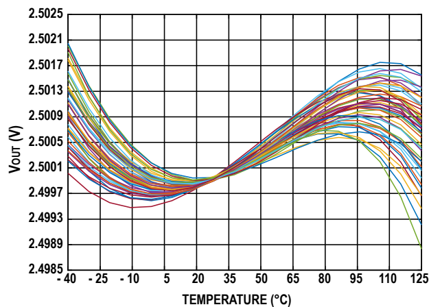
ADR431 温度曲线
