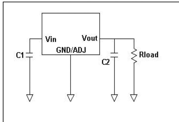
图 1 SPX1117M固定电压版本应用电路
