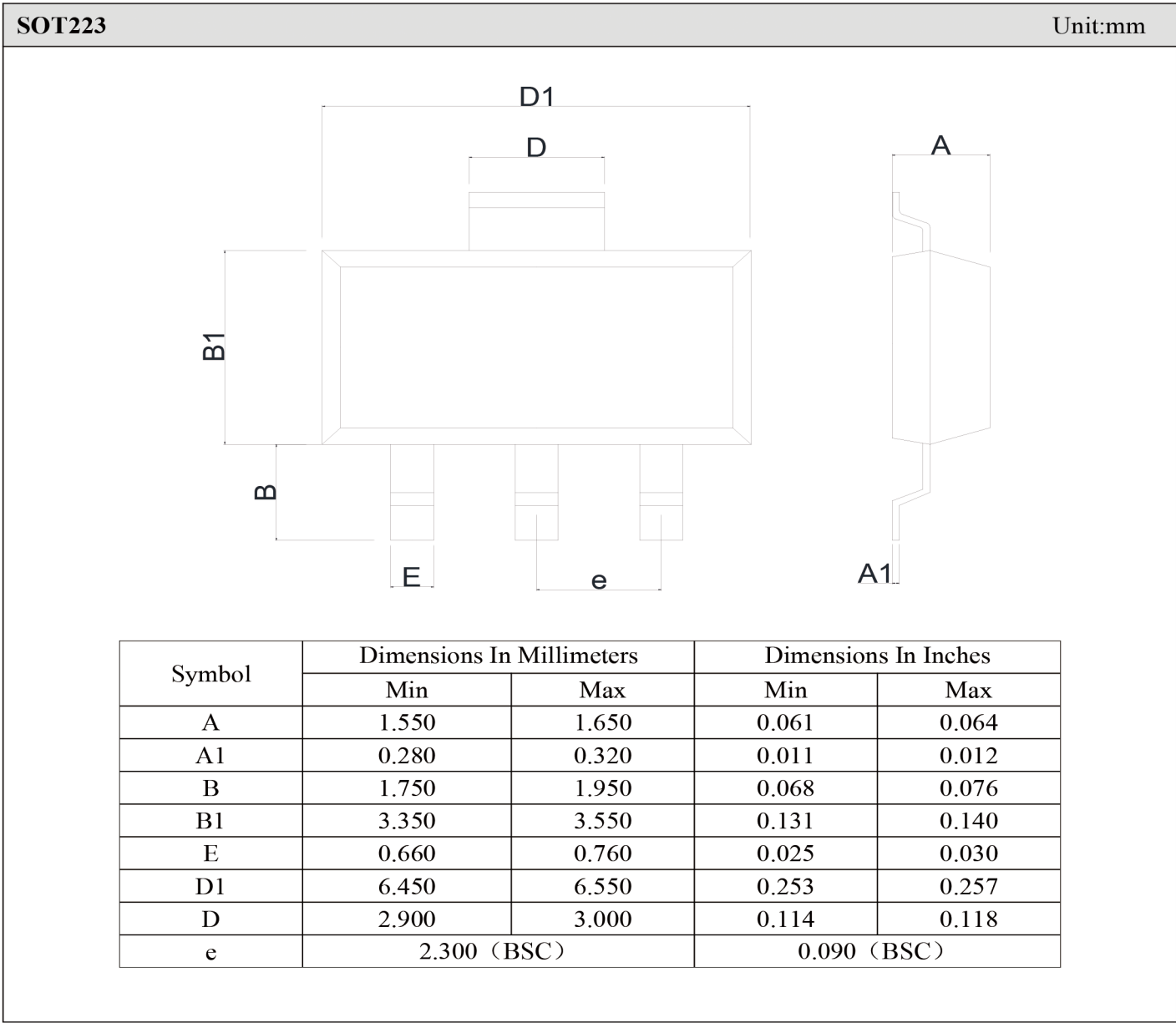
封装外形图:
