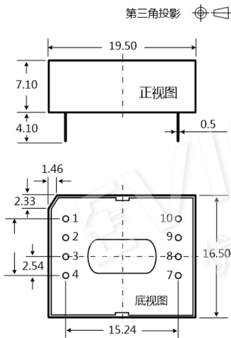
外观尺寸图
