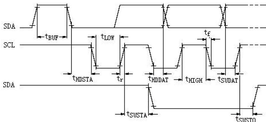
图 4 I 2 C 总线时序波形
