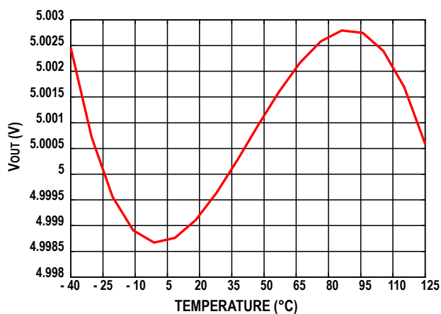
图7. ADR721 典型输出电压与温度关系
