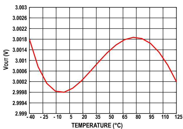
图5. ADR521 典型输出电压与温度关系
