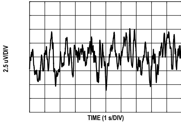
图10. ADR441 输出电压噪声 (0.1 Hz 至 10 Hz)
