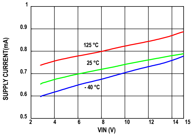
图8. ADR441 输入电流与输入电压的关系
