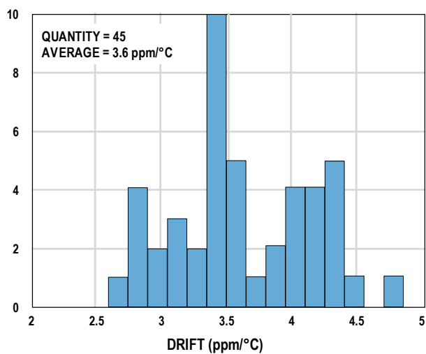
图18. ADR441 温度系数分布图 (MSOP-8 封装)
