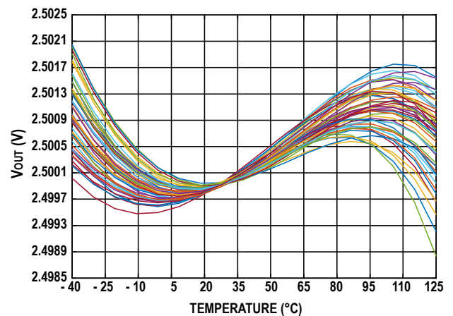
ADR441 温度曲线
