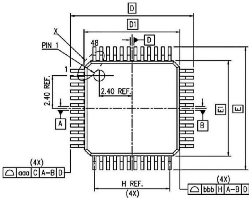
图 18 LQFP48 封装图
