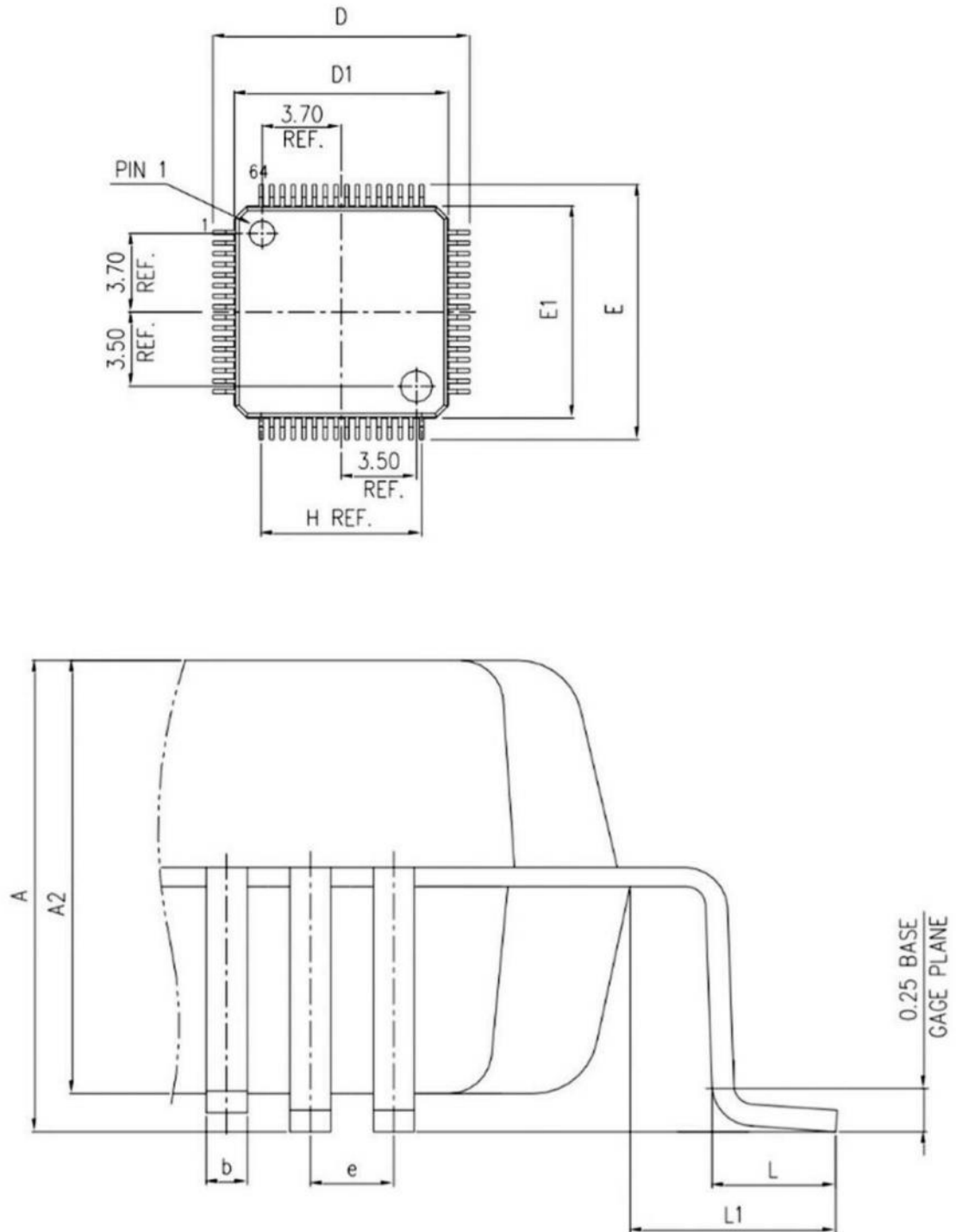
图 15LQFP64 封装图
