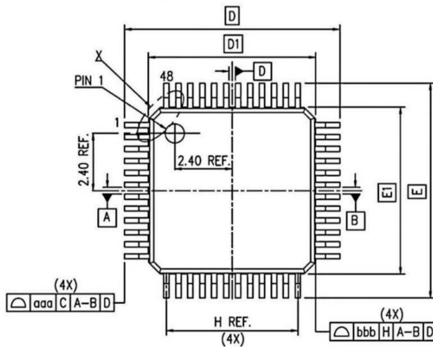
图 18 LQFP48 封装图
