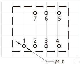
建议印刷图
