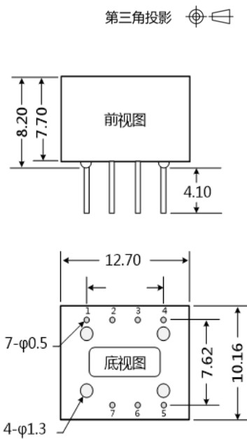
外观尺寸图
