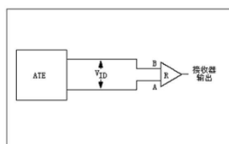
图 10:接收器传播延时测试电路
