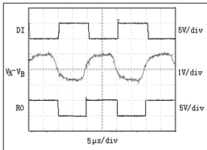
图 12: 在 50kHz 时驱动 4000 英尺的电缆
