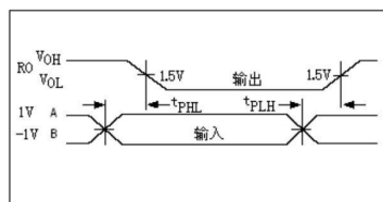
图 8:接收器传播延时
