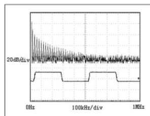
图 11:传输 20kHz 信号时 VP30B3-TB 驱动器输出波形和 FFT 图
