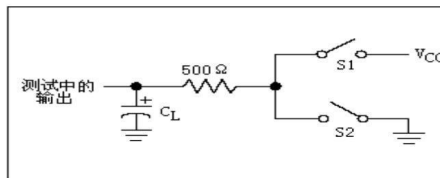
图 5:驱动器使能/无效定时测试负载
