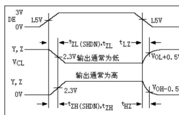
图 7:驱动器使能和无效时间
