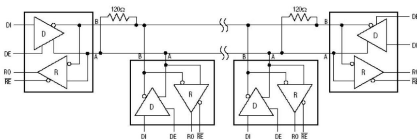
图13: 典型半双工RS-485网络
