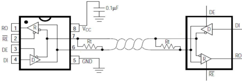
图 1: VP3083-TD 典型半双工应用电路
