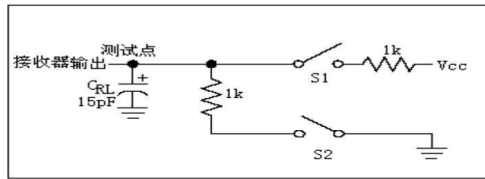
图 3:接收器使能/无效定时测试负载
