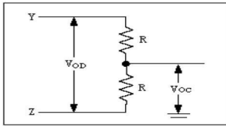
图 2:驱动器 DC 测试负载
