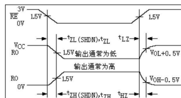
图 9:接收器使能和无效时间
