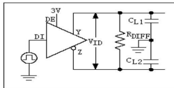
图 4:驱动器定时测试负载
