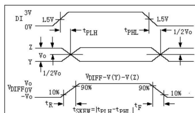
图 6:驱动器传播延时
