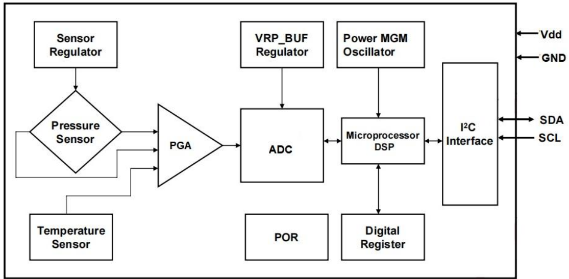
图 1: HBP5013D-2 系列原理框图
