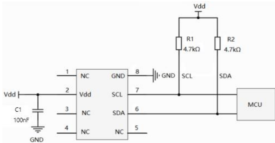
图 4：参考应用电路
