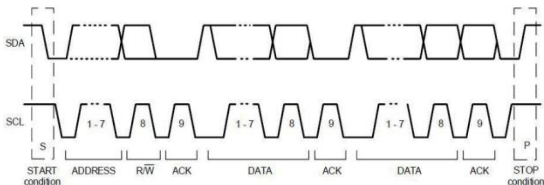
图 3：参考电路 I 2 C 协议数据传输时序图
