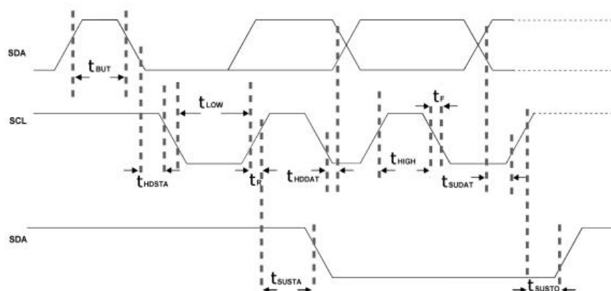
图 2: 参考电路 I 2 C 通讯时序图
