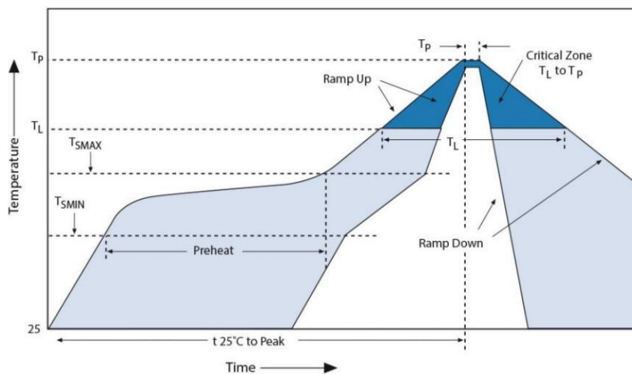
图 7：回流焊温度曲线
