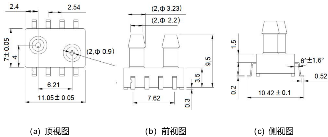
图 5：产品尺寸图
