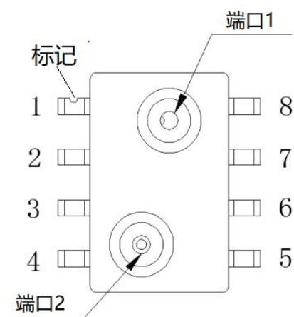
图 6: 引脚定义图
