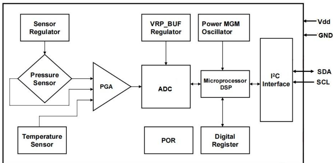
图 1: HBP1412D-2 原理图
