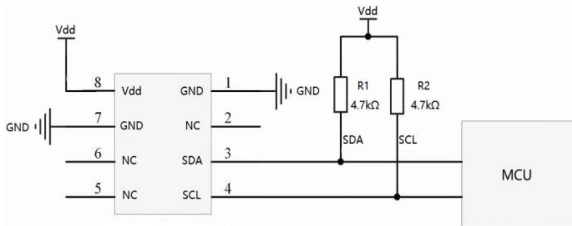
图 4: 参考电路图
