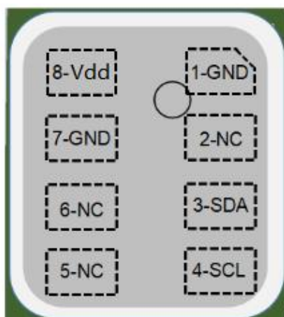
图 11: 引脚定义图 (顶部透视图)
