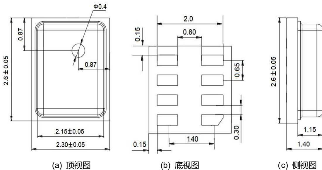
图 5: 封装尺寸图
