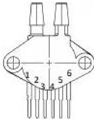
图 6: 引脚定义图
