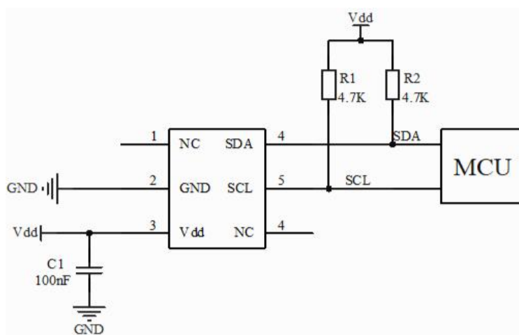
图 4：参考应用电路
