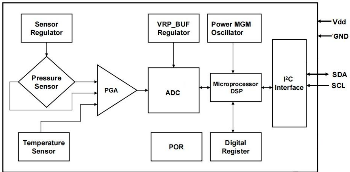
图 1: HBP5033D-2 产品原理框图
