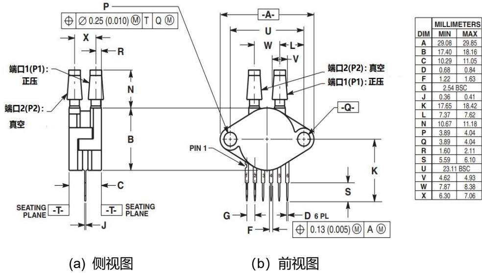
图 5: 产品尺寸图
