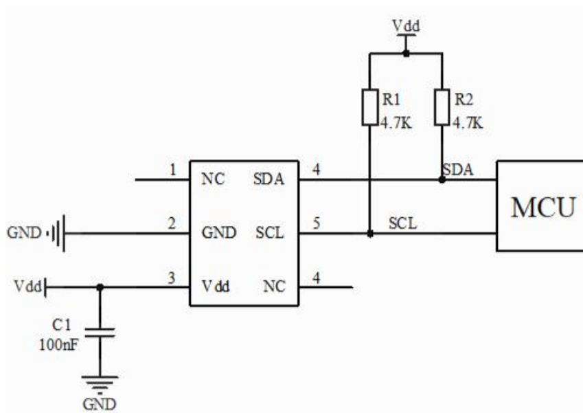
图 4: 参考应用电路
