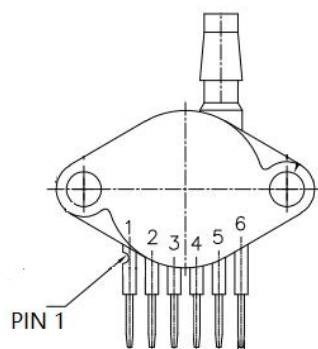
图 6: 引脚定义图
