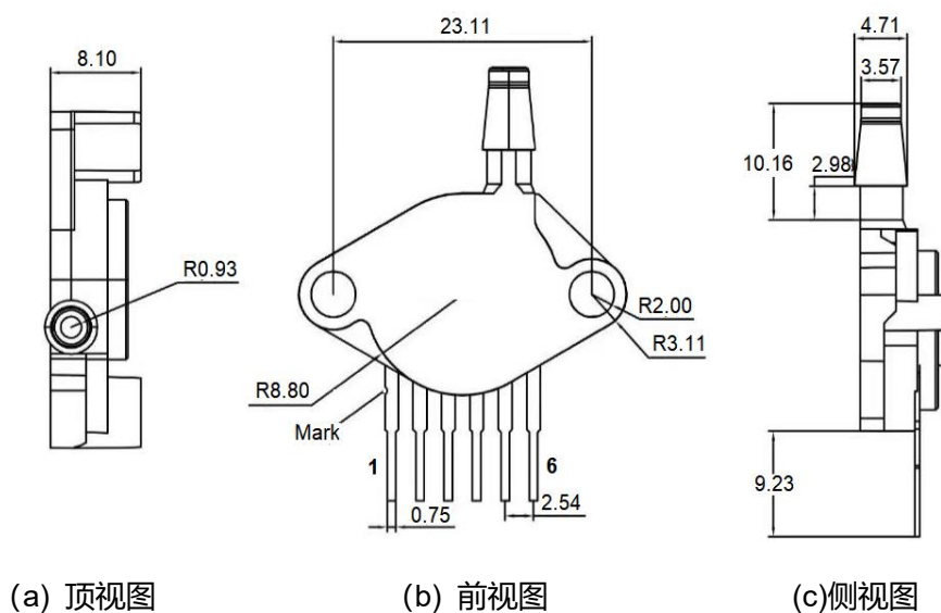
图 5: 封装尺寸图
