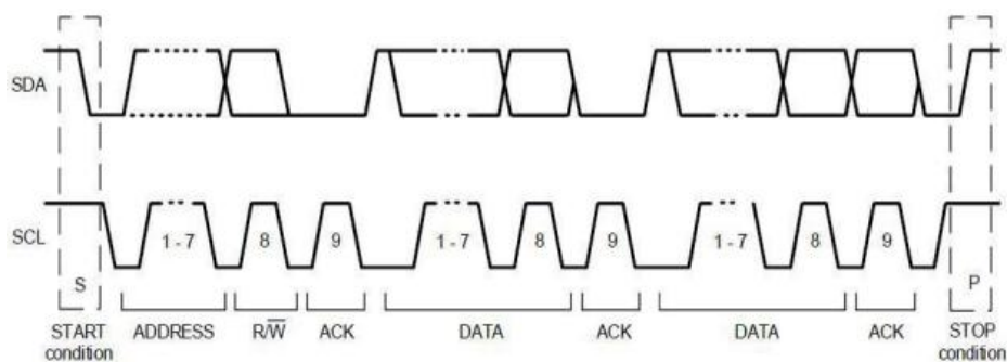
图 3: 参考电路 I²C 协议数据传输时序图
