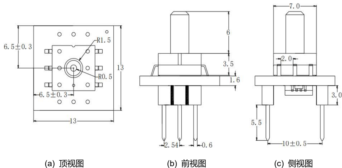
图 5: 封装尺寸图
