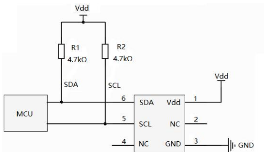
图 4: 参考应用电路
