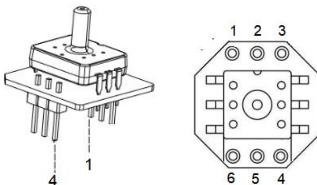
图 6: 引脚定义图
