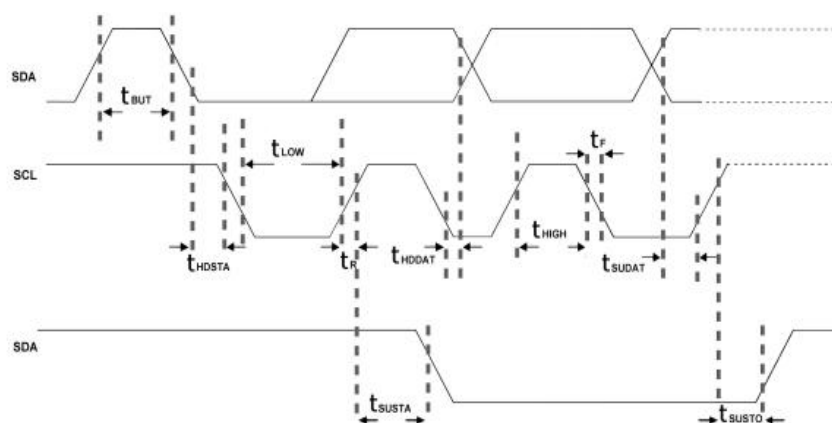
图 2: 参考电路 I 2 C 通讯时序图
