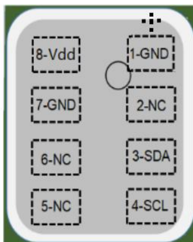
图 6：引脚定义图（顶部透视图）
