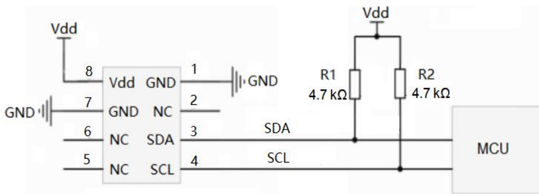
图 4: 参考电路图
