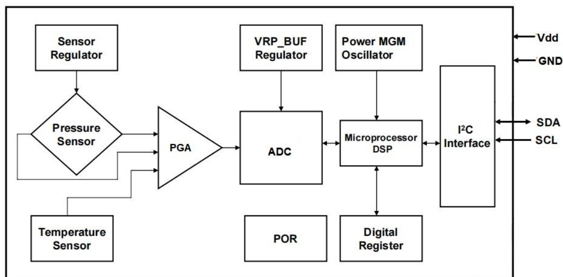
图 1: HBP1402D-2 原理图
