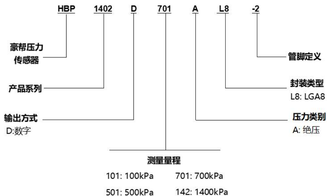
图 8：产品命名规则示意图
