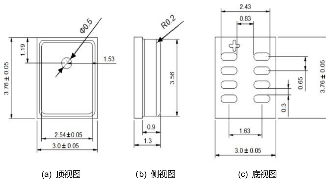
图 5：封装尺寸图
