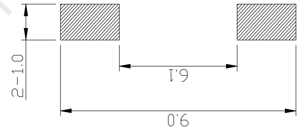
P.C.B LAND DIMENSION
