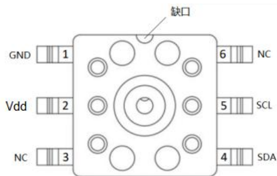
图 6：引脚定义图
