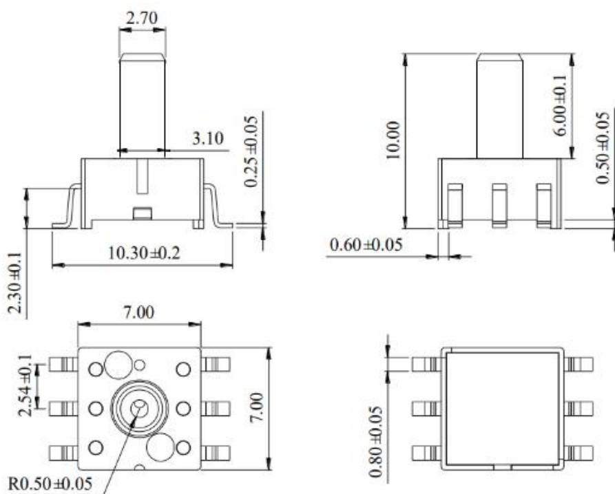
图 5：封装尺寸图
