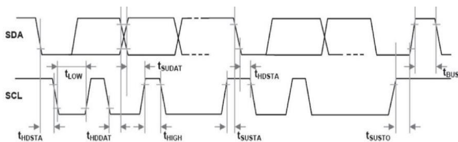
图 3: 参考电路 I²C 协议数据传输时序图
