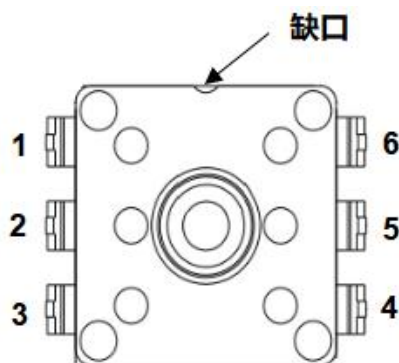
图 6：引脚定义图
