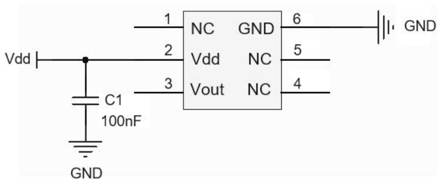
图 3: 参考应用电路
