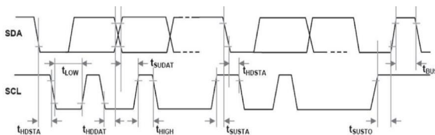
图 3: 参考电路 I 2 C 协议数据传输时序图
