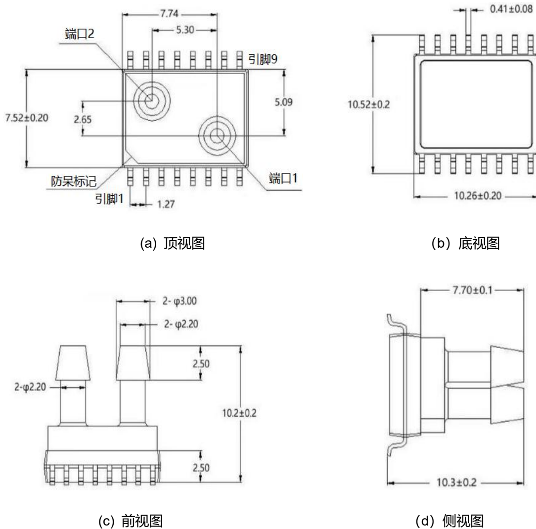
图 5：产品尺寸图
