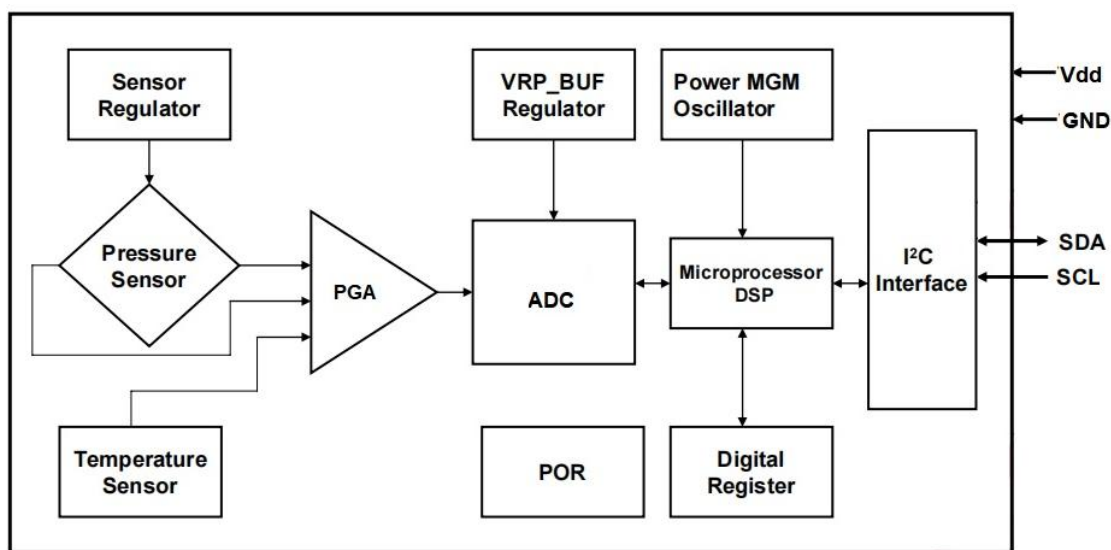
图 1: HBP5003D-2 系列原理框图
