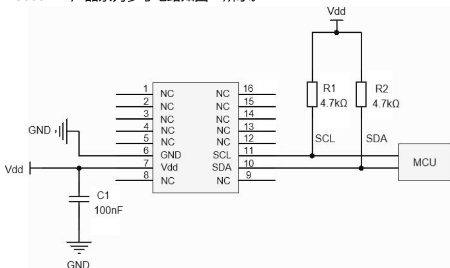
图 4: 参考应用电路
