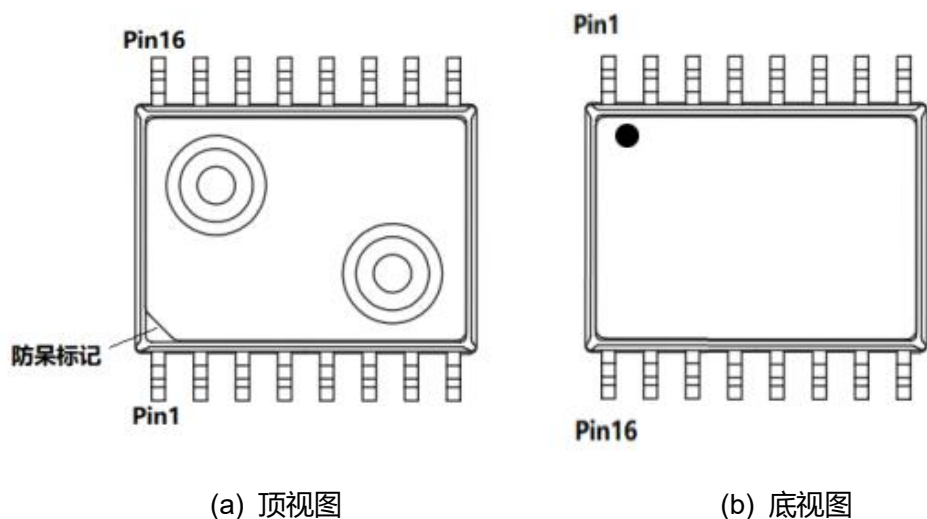
图 6: 引脚定义图
