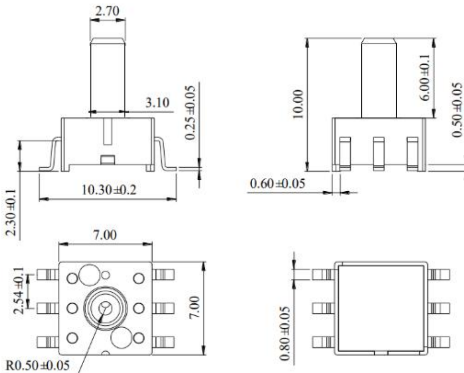
图 1：封装尺寸图
