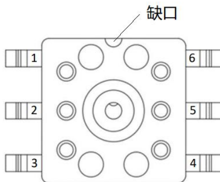
图 2：引脚定义图
