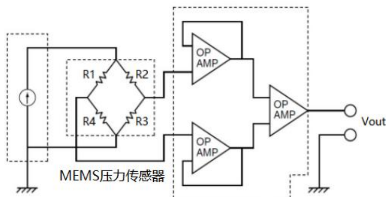
图 3: 参考放大电路
