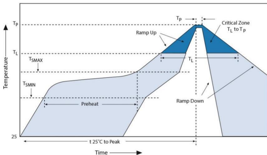
图 4：回流焊温度曲线
