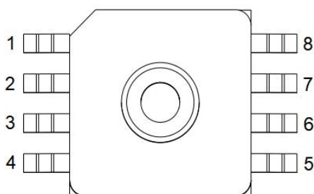
图 2: 引脚定义图
