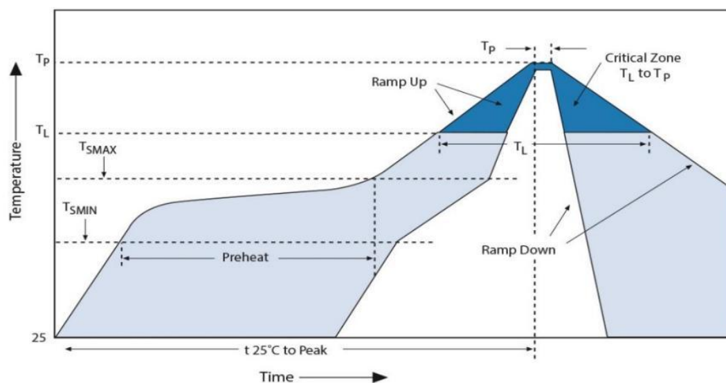
图 4：回流焊温度曲线
