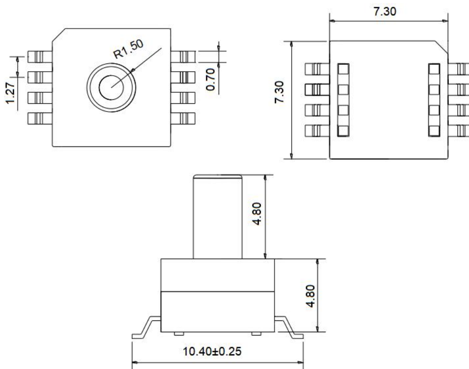
图 1: HBP431 产品尺寸图
