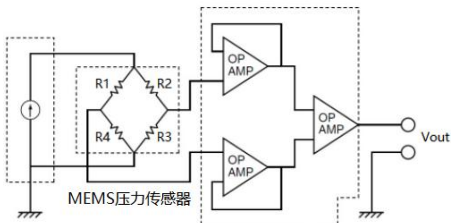
图 3: 参考放大电路
