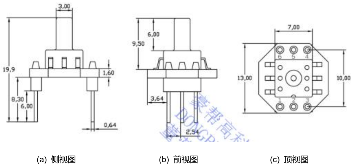
图 4: 封装尺寸图
