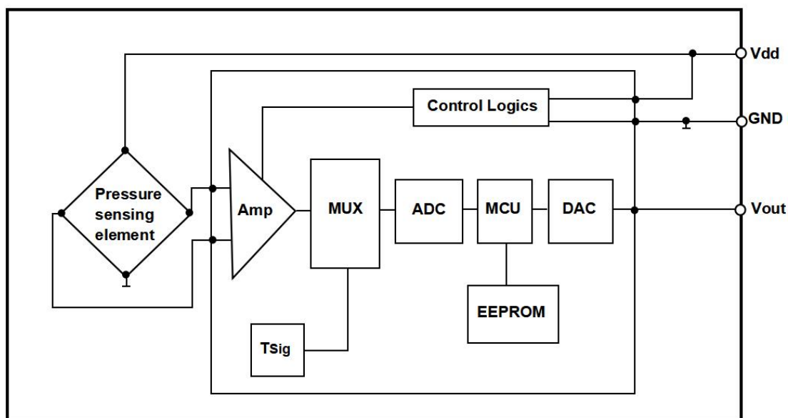
图 1: HBP1901A-2 产品框图
