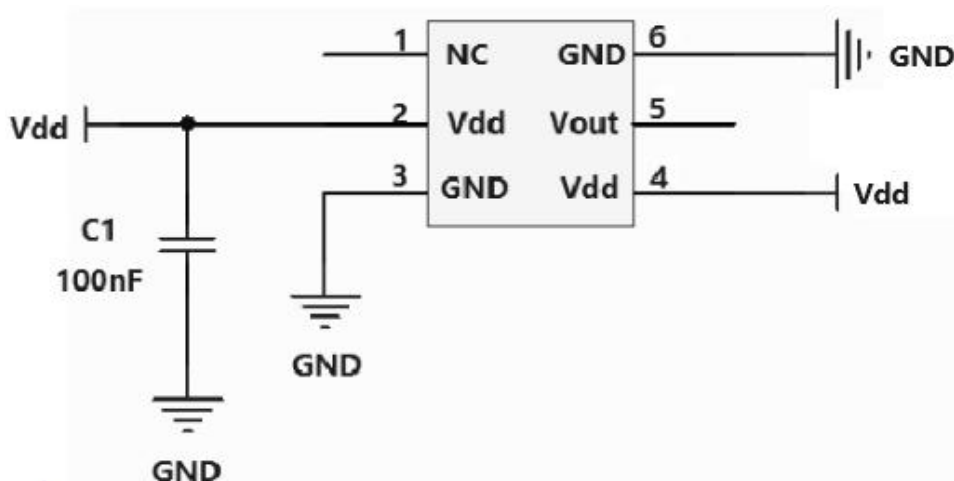
图 3: 参考应用电路
