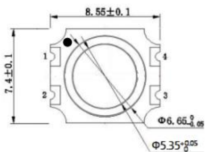
(a) 顶视图
