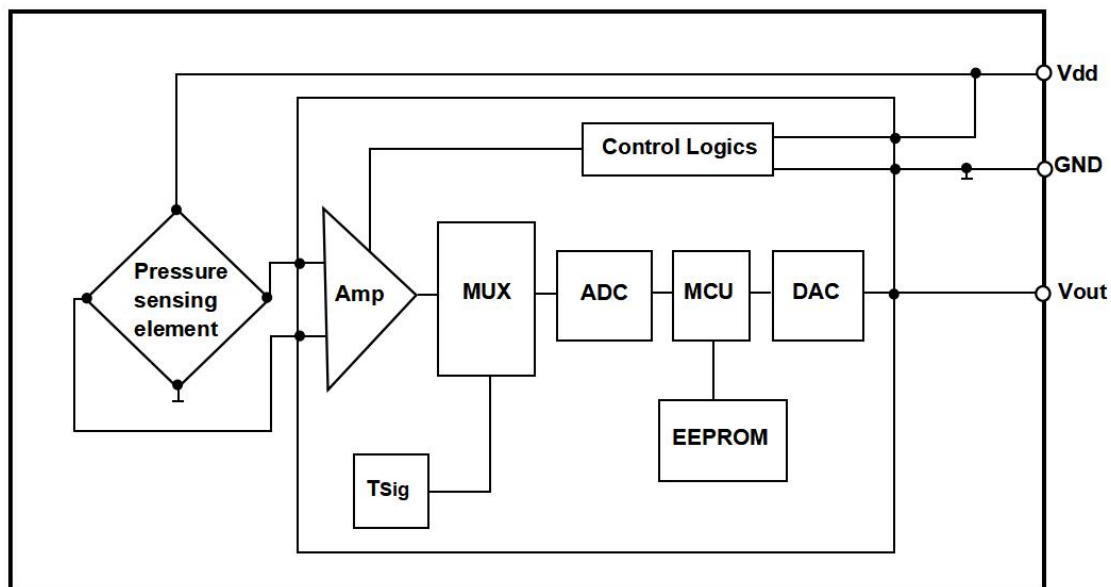
图 1: HBP1822A-P2 产品框图
