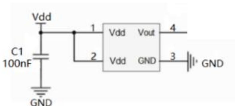
图 3: 参考应用电路
