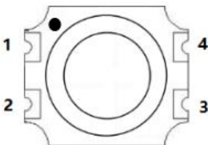
图 5：引脚定义图
