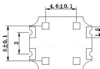
(b) 底视图
