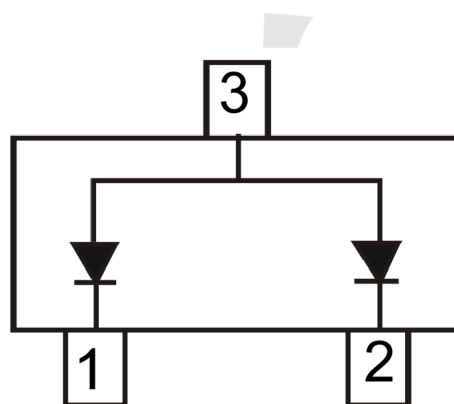
BAS40W-06
